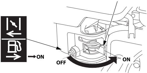
PALANCA DE LA VÁLVULA DE COMBUSTIBLE
